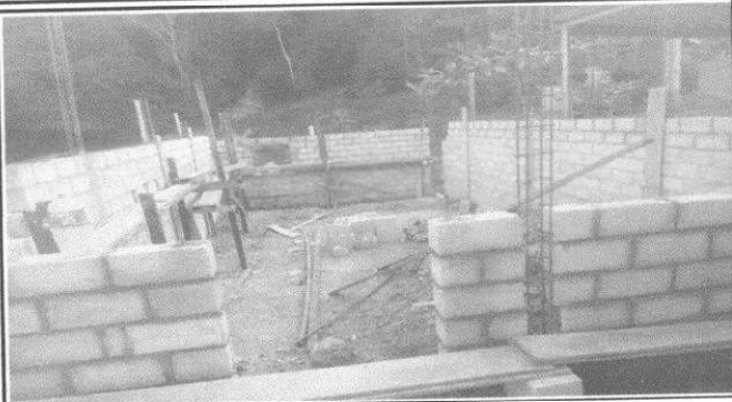
Foto 1: Se observa el inicio de la construcción de la cocina.
